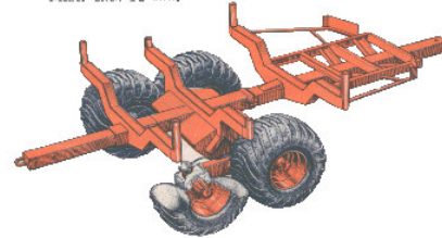
ROSSÖN GRIPLASTARBOGGET LP Max. last 12 ton.
